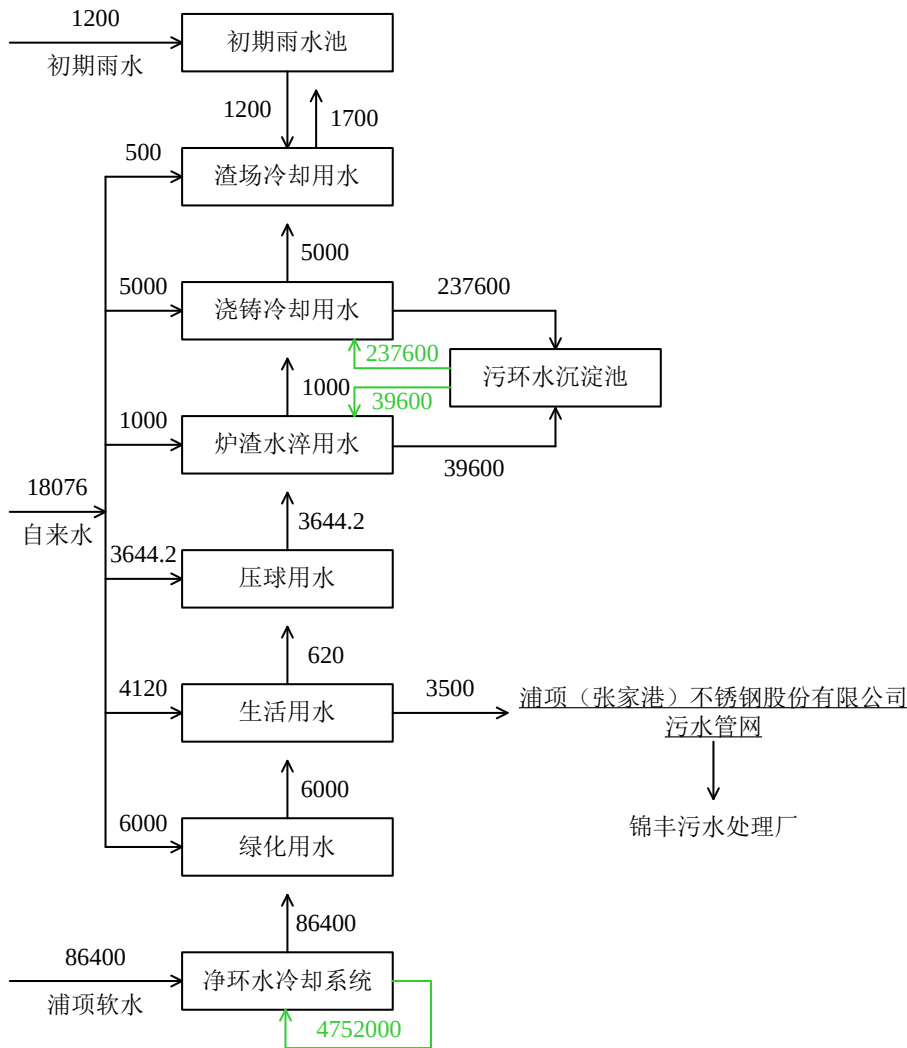
图 4.6-1 本项目建成后全厂水平衡图
