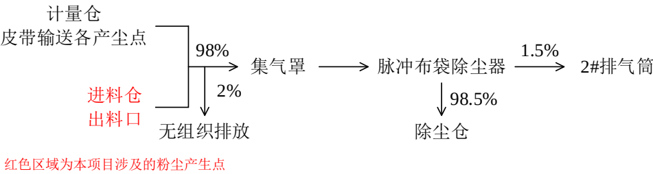
图 7.1-1 物料输送粉尘的处理工艺流程图
