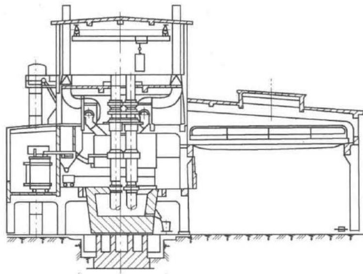
图 3.3-3 矿热炉剖面图
