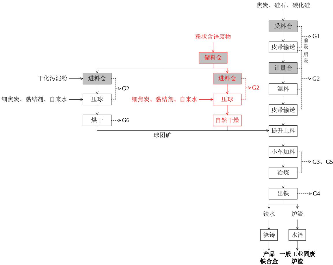
图 4.3-1 危险废物综合利用工艺及产污环节流程图
