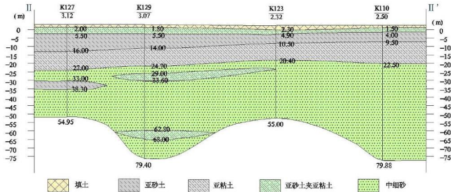
图 6.2-3 厂区水文地质剖面图
